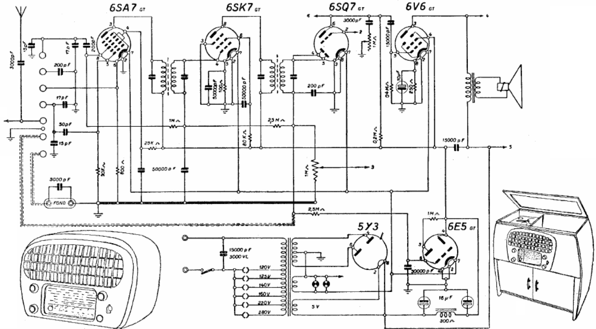
REOM - Sintomagic Radio modd. c1 e c2 - Ricevitori a 10 gamme, con bande espanse, adatti per funzionamento con dispositivo multivox onde ottenere conversazioni bilaterali a viva voce e diffusione in altro ambiente dei programmi radio. (V. schema a parte).
